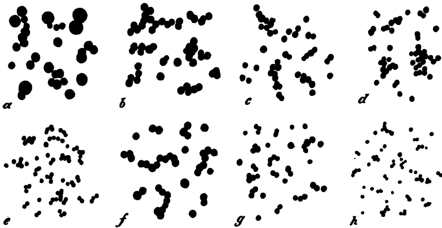
Fig. 4. a-e verschiedene Grösse der Granula, die von dem unverdünnten ALTMANN'schen Gemisch (Osmiumsäure-Kaliumbichromat) aus verschieden starken Lösungen von Deuteroalbumose (schwach sauer reagierend) gefällt werden: a 10-proc., b 3-proc., c 1-proc., d 0,5-proc., e 0,1-proc. Albumose; f-h dieselbe 10-proc. Albumoselösung wie in a , aber mit verdünntem ALTMANN'schen Gemisch gefällt: f \frac{1}{10} , g \frac{1}{50} , h \frac{1}{100} . (Vergr. 600.) Man vergleiche auch die beistehende Tabelle.
